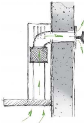
Mauerkasten geöffnet
